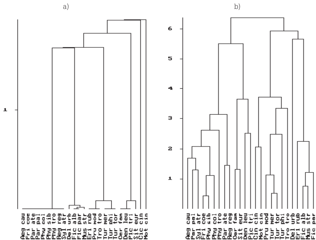
Fig. 2a, b. Porovnanie apriórneho a a posteriorého prístupu na vzorke 25 druhov spoločenstva bukovo-jedľového pralesa, ktoré boli zahrnuté do aposteriórnej analýzy v zmysle štatistických kritérií. Analýza bola štandardizovaná rozpätím hodnôt premenných jednotlivých druhov. Použitá bola metóda nevážených priemerov (UPGMA) a metrika Euklidovských vzdialeností.
